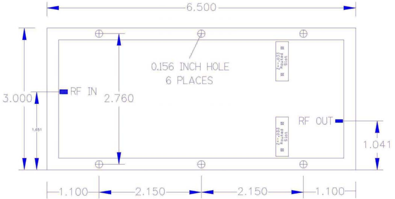
TOP VIEW: P/N UHFTV-25A-40-MH
