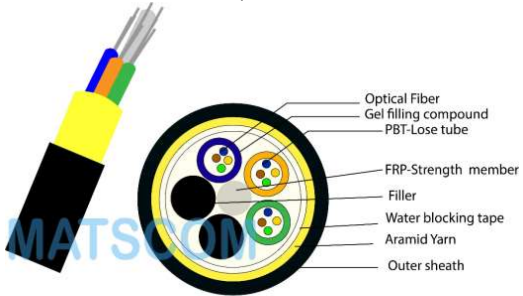
ADSS 12 HILOS
